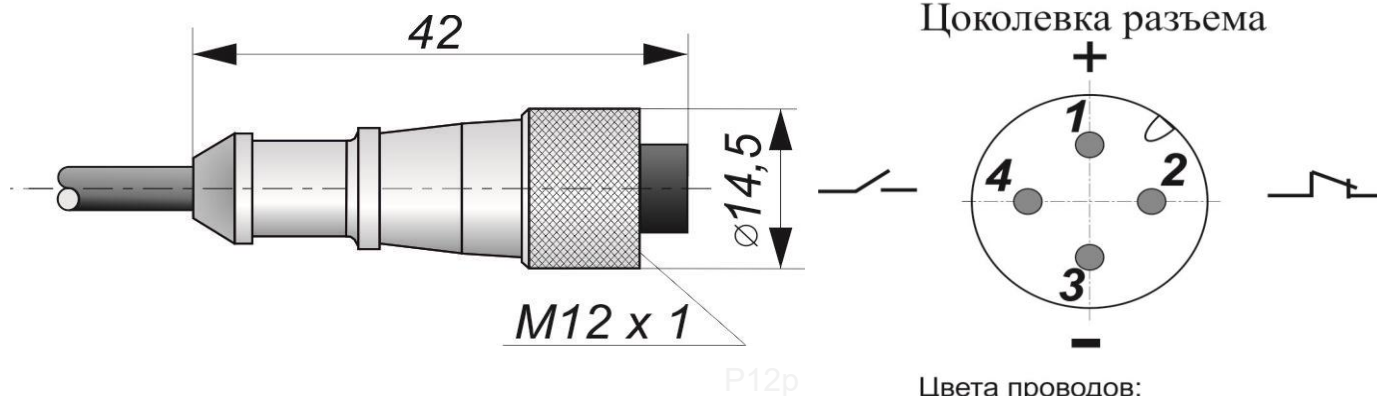
Габаритный чертеж
