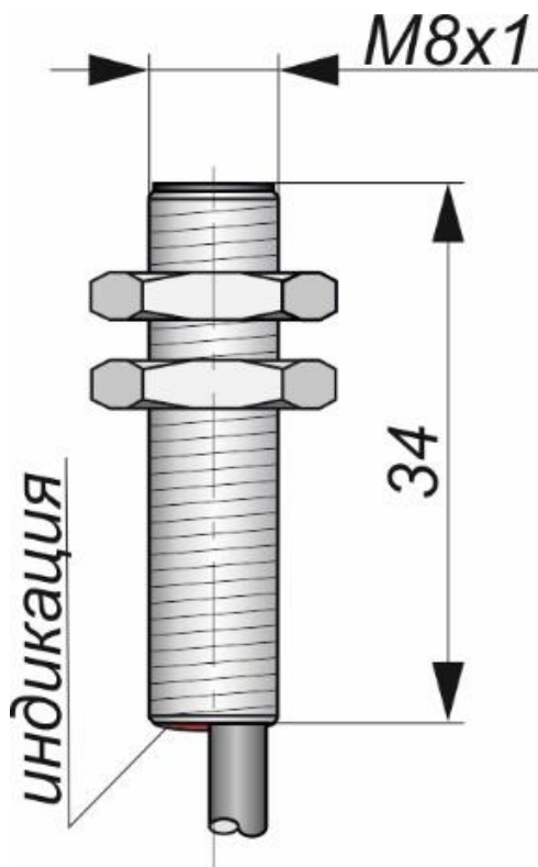
Габаритный чертеж
