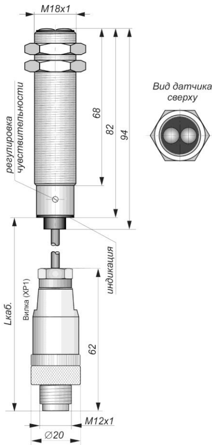
Габаритный чертеж
